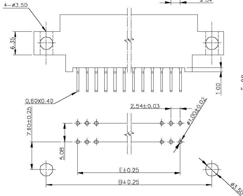
SEC A-A
